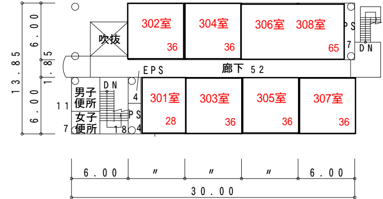
3階平面図 376㎡
